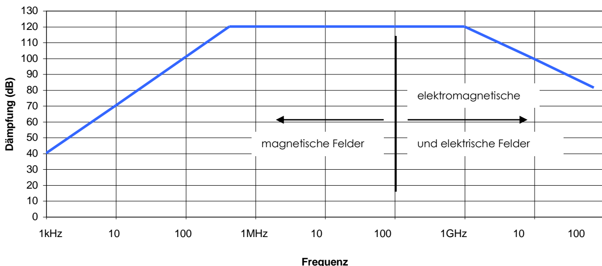
Bild 1 Typische Abschirmdämpfung nach EN 50147-1
